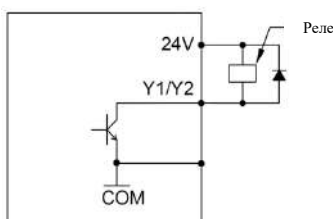
Рис. 3-12 Способ подключения внутреннего источника питания +24 В
