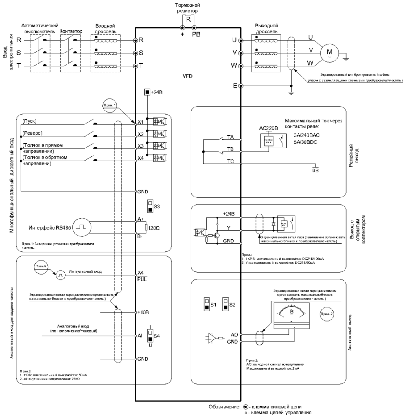
Рис. 3-4. Схема внешних подключений
