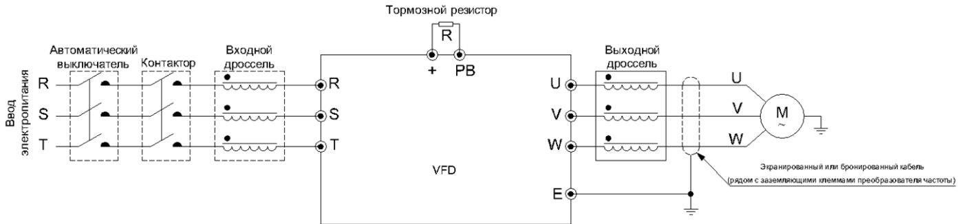
Рис. 3-3.1. Схема подключения преобразователя частоты
