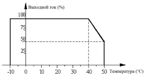
Рис. 2-4. Снижение характеристики преобразователя частоты при превышении допустимой температуры и высоты
