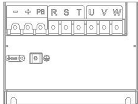
Рис. 3-3.2. Расположение клемм
