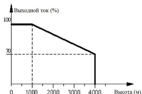
Рис. 2-4. Снижение характеристики преобразователя частоты при превышении допустимой температуры и высоты
