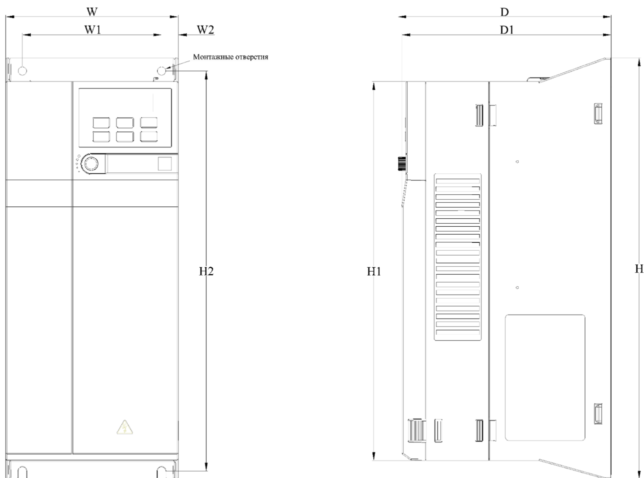
Рис.2-6.3. Чертеж преобразователя частоты типоразмер 3
