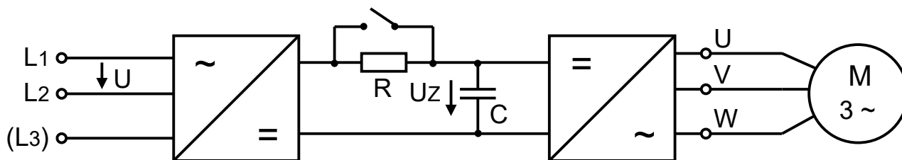
Рис. 1-5. Схема силовой части преобразователя частоты с промежуточным звеном постоянного тока
