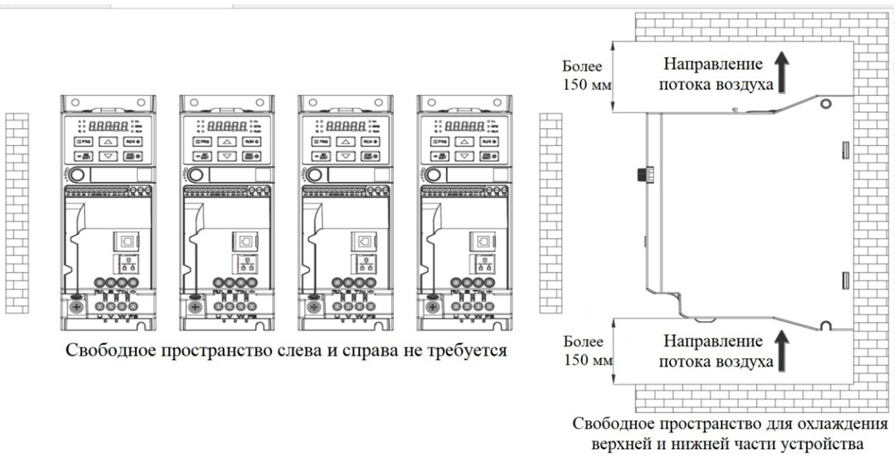
Рис. 2-5. Положение преобразователя частоты и требуемое пространство
