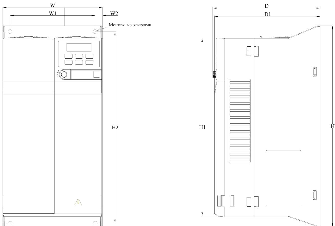
Рис.2-6.4. Чертеж преобразователя частоты типоразмер 1
