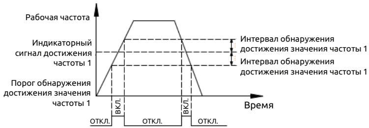
Рис. 7-29 Схема обнаружения достижения заданной частоты
