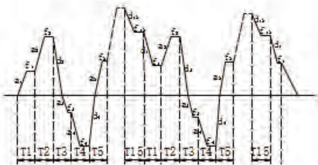
Рис. 7-33 Режим непрерывной работы по программе ПЛК
