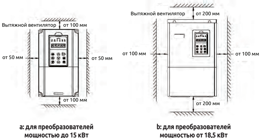
Рис. 3-1 Монтажные размеры
