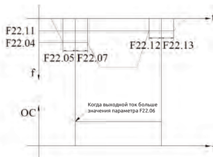
Рис. 7-52. Процесс отпущания тормоза при спуске
