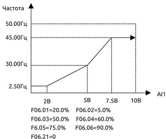
Рис. 7-11 Выбор настройки частоты кривой 1 с использованием входа A1
