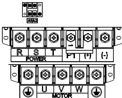
Рис. 4-15 Клеммы силовой цепи для моделей 075G/090P-110G/132P
