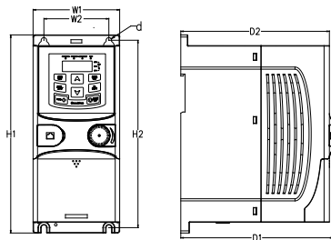
Рис. В-4 Настенный монтаж ПЧ 1ф 220 В/3ф 380 В ( \leq 2,2 кВт) и 3ф 220 В ( \leq 0,75 кВт)
